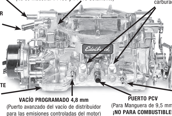
Figura 1 – Ubicaciones de Adaptadores y Puerto de Vacío
