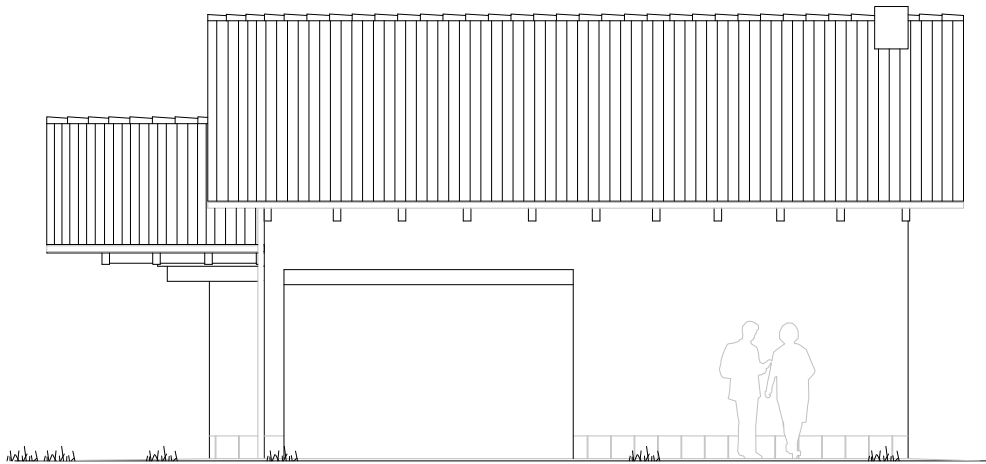
ALZADO POSTERIOR
