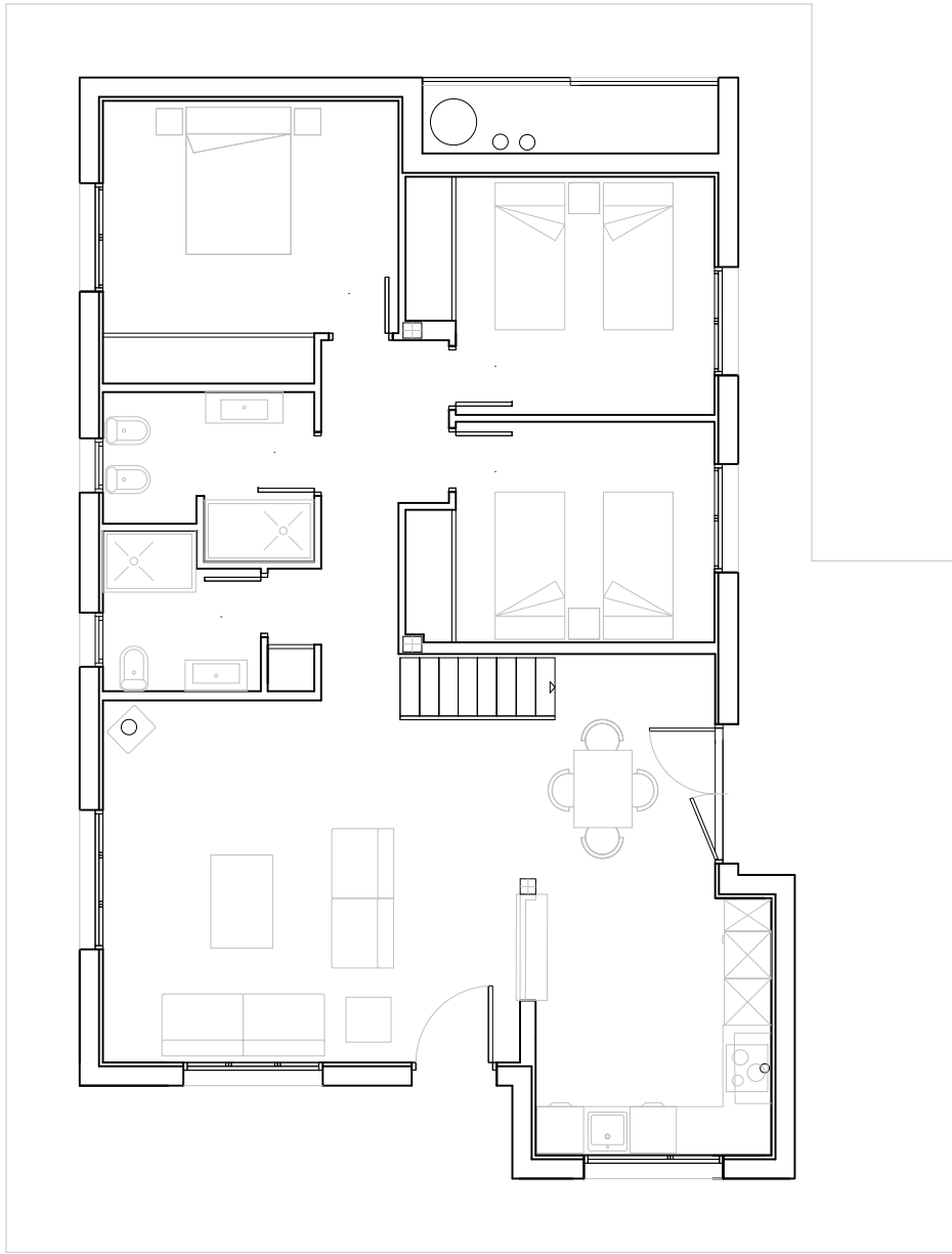
PLANTA BAJA
