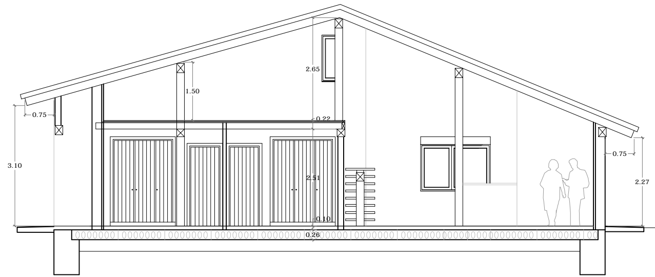
SECCIÓN LONGITUDINAL- 1
