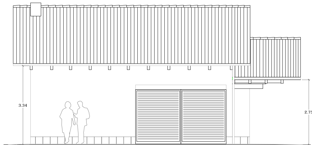
ALZADO OESTE
