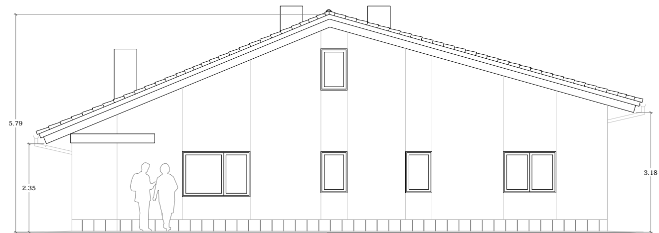
ALZADO NORTE
