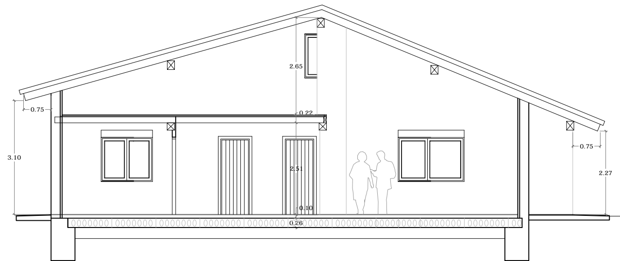
SECCIÓN LONGITUDINAL - 2
