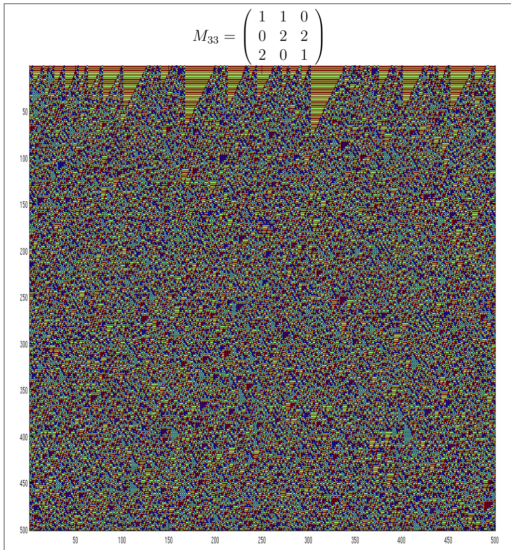
Figura C.18: Simulación de iteraciones de \mu de Bernoulli con distribución \pi = (0,05; 0,9; 0,05) por el AC M_{33}
