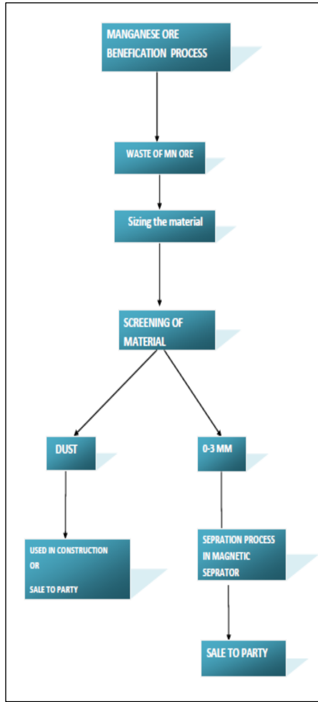
MANGANESE ORE
