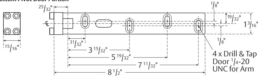
Bottom Pivot Door Portion
