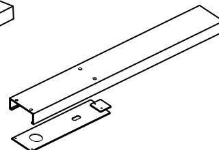
Solid Header (HDS-1750x4500-OHC)
