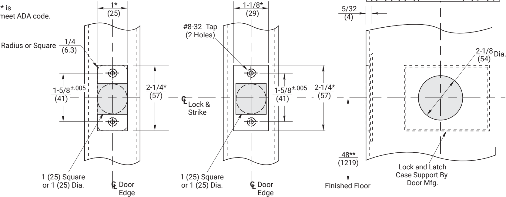
Door Dimensions
