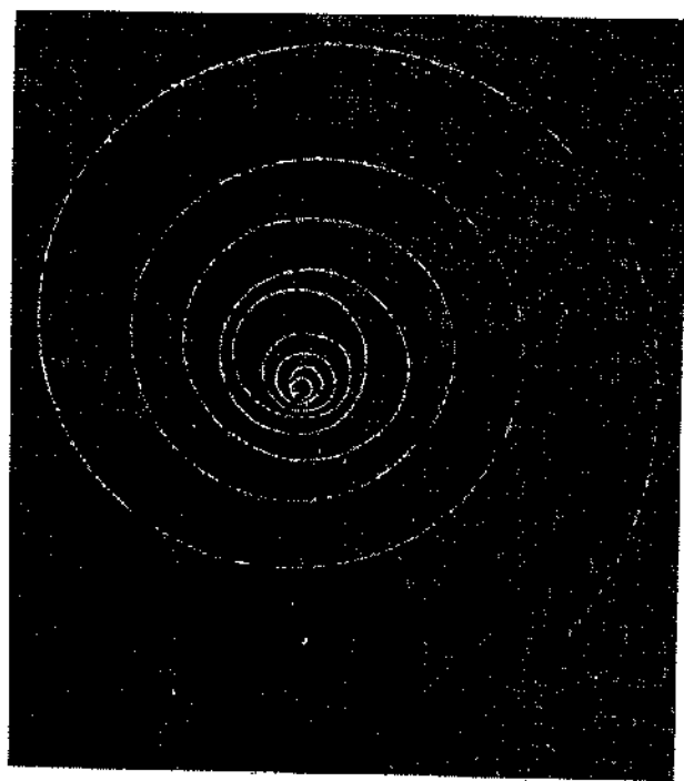
شکل ۱۵. رد یک الکترون در اتاقک حباب هیدروژن مایع. الکترون یک شتاب شعاعی دارد، که ناشی از میدان مغناطیسی است. این شتاب می‌خواهد که مسیر حرکت را دایره‌ای کند. اما الکترون، در اثر برخورد با اتمهای هیدروژن، کند می‌شود. بنابراین، یک شتاب مماسی هم دارد. مسیر حاصل از این دو شتاب، مارپیچ است.
