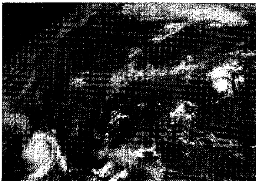
شکل ۱۸. مرکز کم فشاری بر زمین چرخان. با جریان بافتن هوا به طرف مرکز، ناظر ناخست در نیمکره شمالی می بیند که هوا در جهت پادساعتگرد می چرخد. گردباد (عکس سمت راست) چنین مرکز کم فشاری است.
