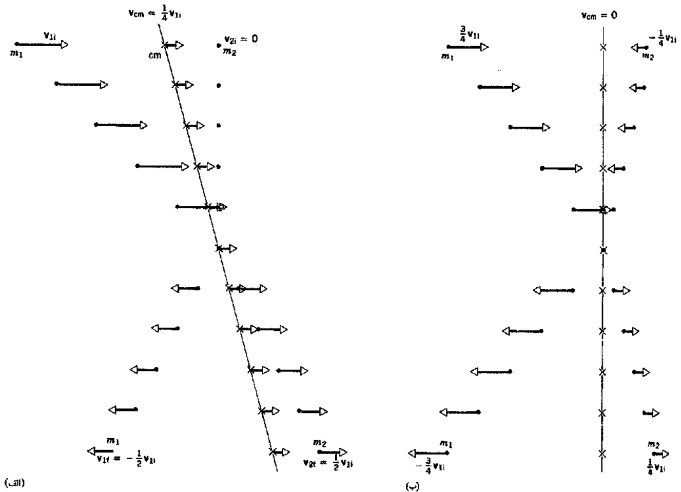
شکل ۱۶. یک رشته "تصویرهای لحظه‌ای" مربوط به دو ذره یا جرمهای m_1 و m_2 = 3m_1 که به‌طور کشسان در یک‌بعد با هم برخورد می‌کنند. مرکز جرم دو ذره با علامت \times مشخص شده است. (الف) چارچوب مرجع آزمایشگاه. (ب) چارچوب مرجع مرکز جرم.
