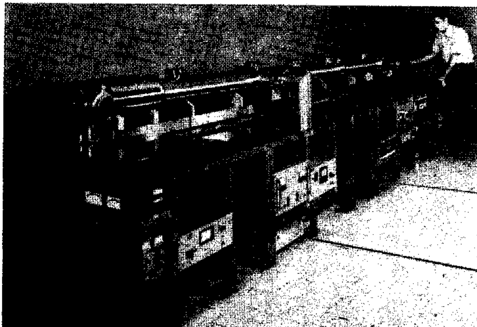
شکل ۱. استاندارد پسماد اتمی (سزیم) شماره NBS-۶ در مؤسسه ملی استانداردها و تکنولوژی در بولدر کلرادو. این استاندارد اصلی یکای زمان در ایالات متحد امریکا است.
