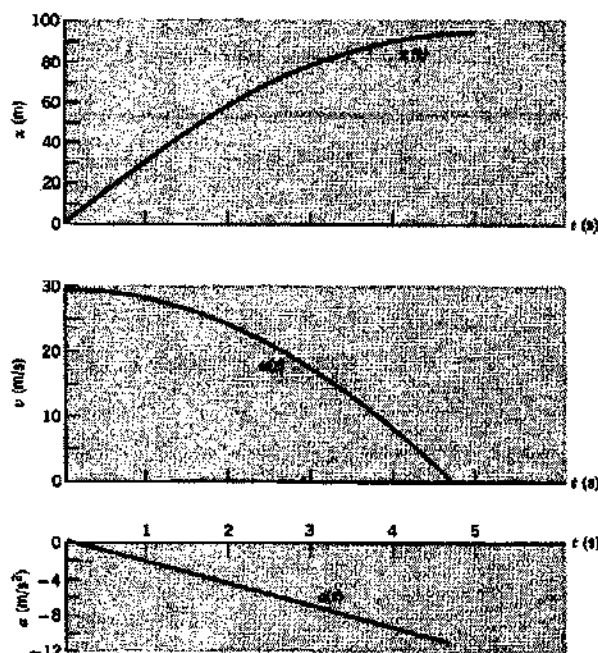
شکل ۱۱. مثال ۴. x(t) و v(t) حاصل از a(t) ، که به طور خطی با زمان تغییر می‌کند.
