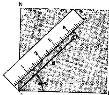
شکل ۲. بردار d نشان‌دهنده یک جابه‌جایی به اندازه 42m (در مقیاس 1cm = 10m ) در جهت 45^\circ شمال شرقی است.
