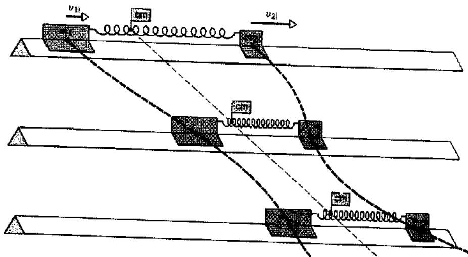
شکل ۲. به دو جسم لغزنده که توسط فنر کشیده شده‌ای به هم متصل شده‌اند سرعت‌های اولیه دلخواهی داده شده است. این دو جسم حرکات پیچیده‌ای دارند، در حالی که مرکز جرم که با پرچم مشخص شده است با سرعت ثابت حرکت می‌کند. بازه‌های زمانی بین وضعیت‌های متوالی، با هم مساوی‌اند.
