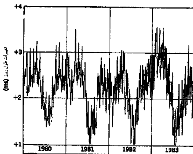
شکل ۲. تغییرات طول روز در یک دوره ۴ ساله. دقت کنید که مقیاس عمودی تنها ۳ms = ۰.۰۰۳s است. ۱
