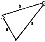
شکل ۴. جمع برداری a + b = s . این شکل را با شکل ۱ ج مقایسه کنید.
