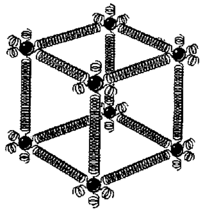
شکل ۱۱. اتصالات یک جسم جامد روی یک شبکه سه‌بعدی تکرارشونده توزیع شده‌اند. نیروهای بین اتمی را با قطر نمایش داده‌ایم.
