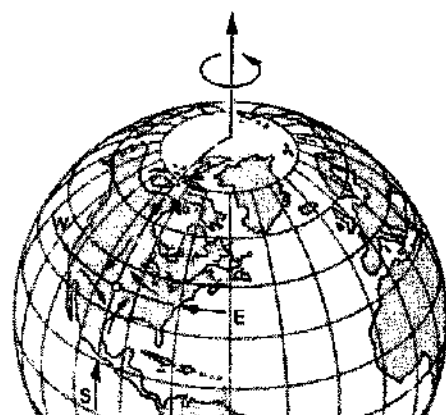
شکل ۱۸. مرکز کم فشاری بر زمین چرخان. با جریان بافتن هوا به طرف مرکز، ناظر ناخست در نیمکره شمالی می بیند که هوا در جهت پادساعتگرد می چرخد. گردباد (عکس سمت راست) چنین مرکز کم فشاری است.
