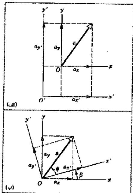
شکل ۱۰. (الف) مبدأ O دستگاه مختصات شکل ۱۰الف به نقطه O' رفته یا منتقل شده است. مؤلفه‌های x و y بردار a با مؤلفه‌های x' و y' آن برابرند. (ب) محورهای x و y به اندازه زاویه \theta چرخیده‌اند. مؤلفه‌های x' و y' با مؤلفه‌های x و y متفاوت‌اند (دقت کنید که مؤلفه y' در این مورد از مؤلفه x' کوچکتر است، در حالی که در شکل ۱۰الف مؤلفه y از مؤلفه x بزرگتر بود)، اما بردار a عوض نشده است. محورهای مختصات را به اندازه چه زاویه‌ای باید چرخاند تا مؤلفه y' صفر شود؟
