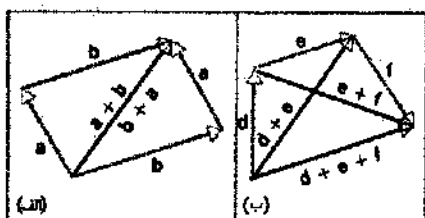
شکل ۴. (الف) قانون جابه‌جایی جمع برداری: a + b = b + a . (ب) قانون شرکت‌پذیری جمع برداری: d + (e + f) = (d + e) + f .
