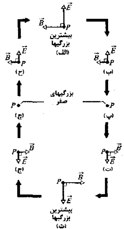
شکل ۲۹-۴ (الف) - (ح) تغییرات میدان الکتریکی \vec{E} و میدان مغناطیسی \vec{B} در نقطه دور P در شکل ۲۹-۳ وقتی که یک طول موج از موج الکترومغناطیسی از آن می‌گذرد. در این شکل، موج مستقیماً به سمت خارج صفحه حرکت می‌کند. بزرگی و جهت این دو میدان به طور سینوسی تغییر می‌کنند. توجه کنید که آنها همواره بر یکدیگر و بر جهت حرکت موج عمودند.
