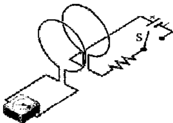
شکل ۲۶-۲ درست وقتی کلید S وصل (۱:۰) جریان در حلقهٔ سمت راست برقرار شود، با کلید قطع شود (تا جریانی در حلقهٔ سمت راست قطع شود) آمپرسنج در حلقهٔ سمت چپ جریانی را نشان می‌دهد. حلقه‌ها هیچ حرکتی ندارند.
