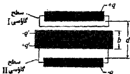
شکل ۱۸-۲۱ یک خازن تخت شامل تیفه‌ای دی الکتریک است که فقط بخشی از فضای میان صفحه‌ها را پرمی کند.
