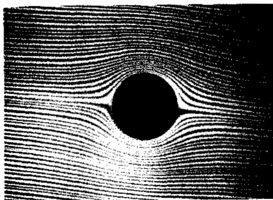
شکل ۱۶-۳۰ شارش پایانی یک شار در اطراف یک استوانه که به وسیله یک ردیاب رنگی ایجاد شده است.
