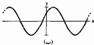
شکل ۳۲-۷ (یک موج سینوسی پیشرونده در t=0 با ثابت فاز \phi (الف) و (ب) \pi/\text{rad} )
