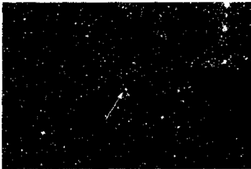
شکل ۱۱-۴۳ (الف) ستاره‌ای موسوم به سندولیک ۱ که در سال ۱۹۸۷/۱۳۶۶ پدیدار شد. (ب) سپس شروع به دریافت نور از ابرنواختر آن ستاره کردیم، که به آن نماد SN1987a تخصیص داده شده است؛ این انفجار، ۱۰۰ میلیون بار درخشانتر از خورشید ما بود و می‌توانست با چشم غیر مسلح دیده شود. این انفجار در فاصله ۱۵۵۰۰۰ سال نوری دور از ما رخ داده و بنابراین در واقع ۱۵۵۰۰۰ سال پیش روی داده است.
