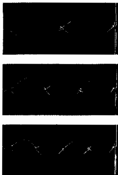
شکل ۲۲-۳۲ عکسهای استروبوکوپی، نقشهای موج ایستاده (ناقص) را در ریسمانی که یک ارتعاش کننده در انتهای چپ آن را به نوسان واداشته است، آشکار می‌کند. این نقشها در بسامدهای معینی از نوسان پیش می‌آیند.
