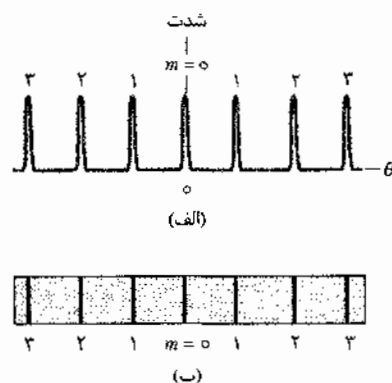
شکل ۳۶-۱۹ (الف) نمودار شدت حاصل شده از یک توری پراش با شیارهای خیلی زیاد شامل قله‌های باریکی است که با مرتبه m آنها نشان داده شده‌اند. (ب) فریزهای روشن متناظر روی صفحه مشاهده خط نامیده می‌شوند و در اینجا نیز با عددی m نشانه‌گذاری شده‌اند.
