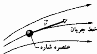
شکل ۱۵-۳۰ یک عنصر شار به هنگام حرکت یک خط جریان را تشکیل می‌دهد. بردار سرعت عنصر در هر نقطه بر خط جریان مماس است.
