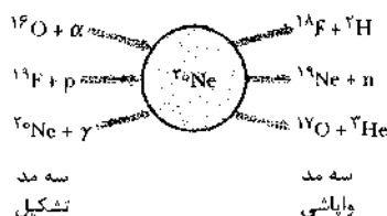
شکل ۱۴-۴۲ مدهای تشکیل و مدهای واپاشی هسته مرکب ^{20}\text{Ne}
