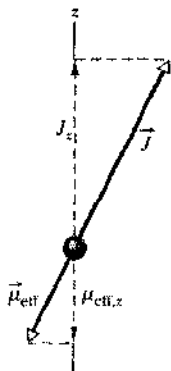
شکل ۷-۴۰ مدل کلاسیکی که بردار اندازه حرکت زاویه‌ای کل \vec{J} و بردار گشتاور مغناطیسی مؤثر \vec{\mu}_{\text{eff}} را نشان می‌دهد.
