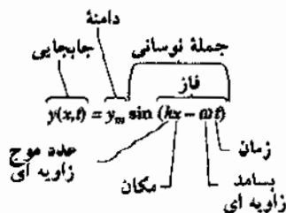
شکل ۳۲-۴ نام کمیت‌های معادله ۳۲-۲ برای یک موج سینوسی عرضی
