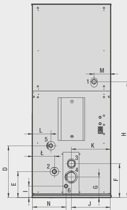
Widok z tyłu BIOPELLET PRO 8
