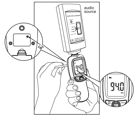
Rysunek 1 ( Schemat kalibracji źródła dźwięku )
