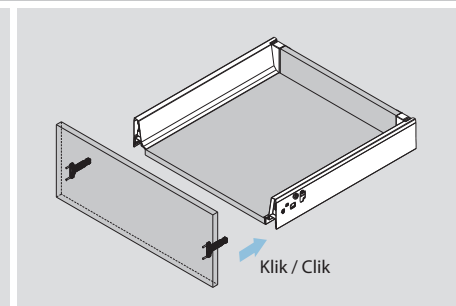
Montaż spodu / Bottom assembly
