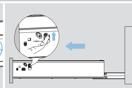
Podnieś uchwyt zwalniający i wyciągnij szufladę Lift the release handle and pull out the drawer
