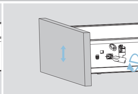
Regulacja góra - dół Up & down adjustment
