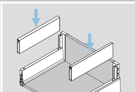
Montaż boków / Side assembly
