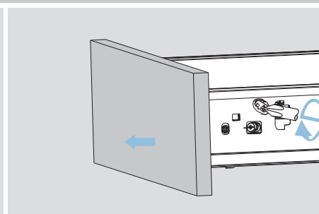
Obróć śrubokręt, aby zwolnić przód szuflady Turn screw driver to release the drawer front
