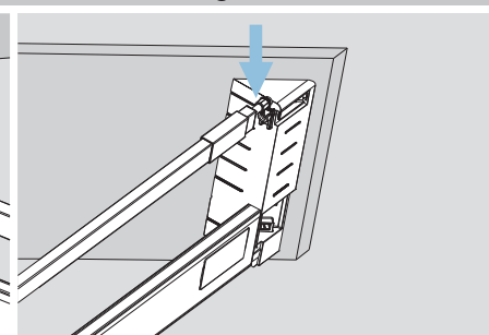
Montaż frontu / Front assembly
