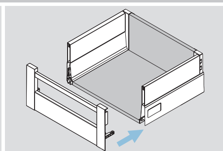
Montaż frontu / Front assembly Klik / Click
