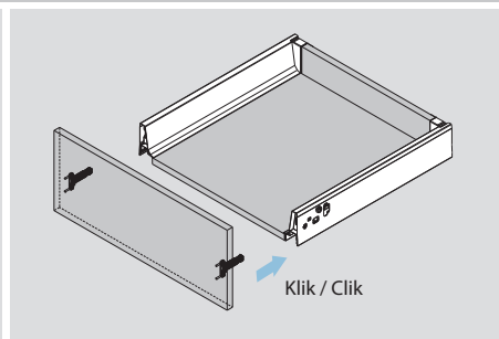
Montaż tyłu / Back assembly
