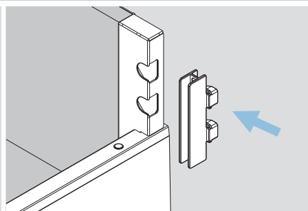
Montaż tylnej ścianki / Back assembly
