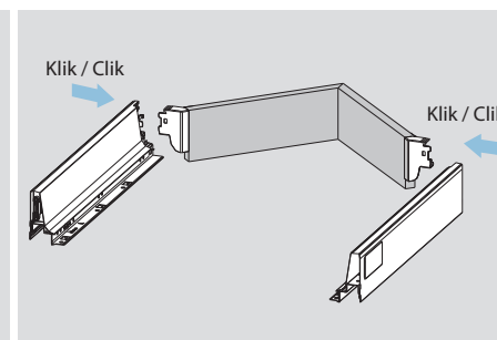
Montaż boków / Side assembly Klik / Click
