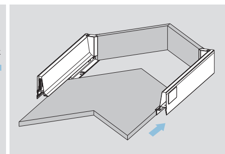
Montaż spodu / Bottom assembly
