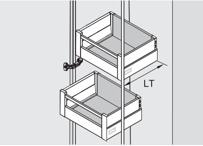
LT= Głębokość nominalna korpusu / Internal cabinet depth
