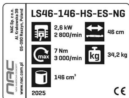
Tabliczka znamionowa
