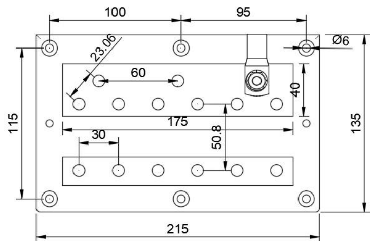
SZYNA DODATNIA
