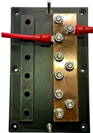
SZYNA UJEMNA
