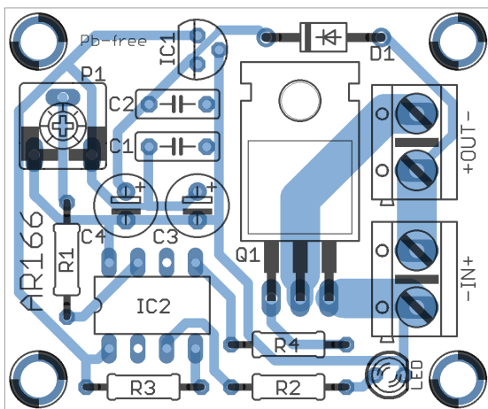
Rys. 2. Schemat montażowy
