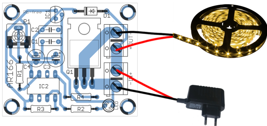
Rys. 3. Przykład podłączenia
