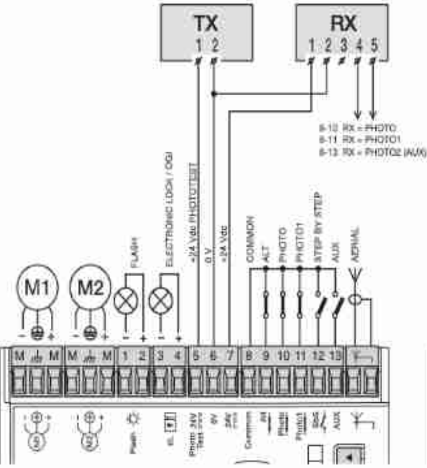
C Połączenie: bez użycia „Stand-By wszystko” z „Fototestem”
