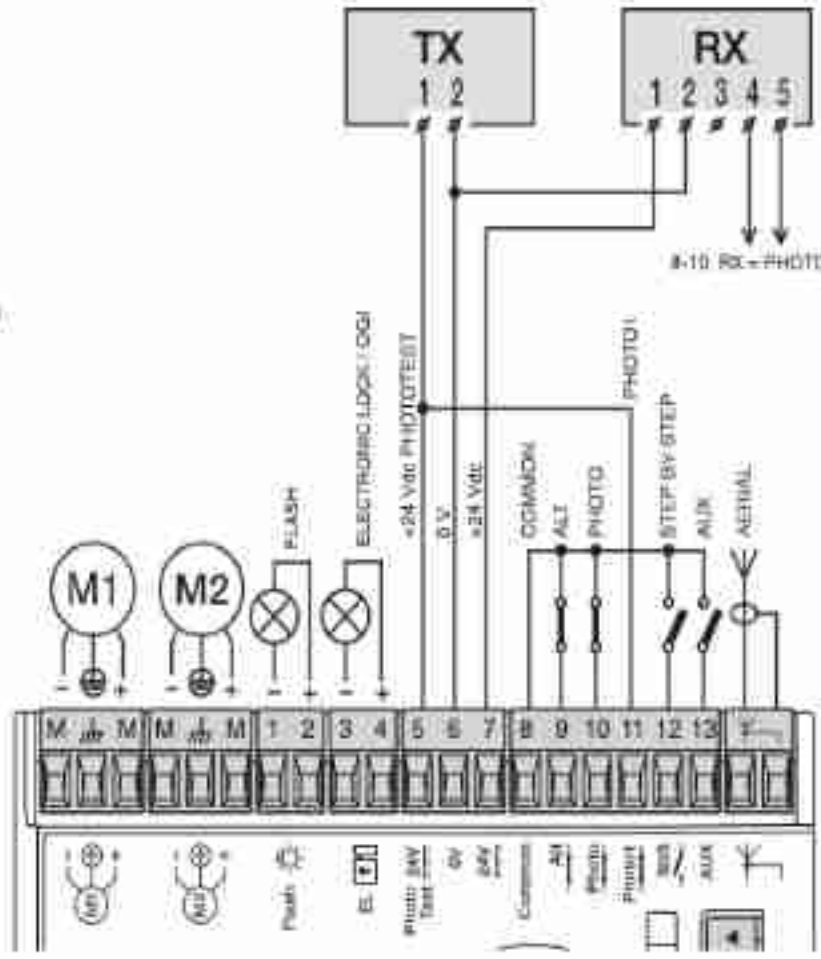
D Połączenie: bez użycia „Stand-By wszystko” z „Fototestem” i bez „Photo1”
