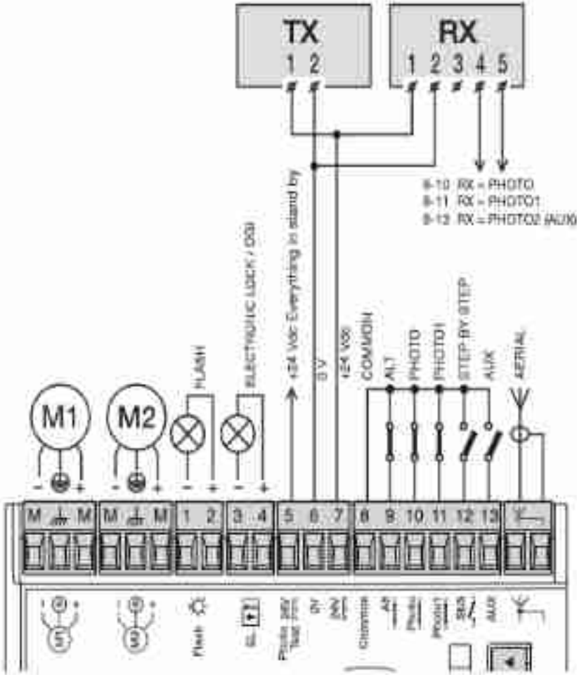
B Standardowe połączenie: bez użycia „Stand-By wszystko” i bez „Fototestu”
