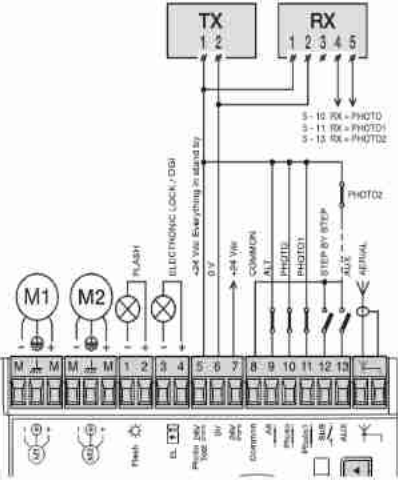
A Połączenie z aktywnym „Stand-By wszystko” (oszczędzanie energii)
