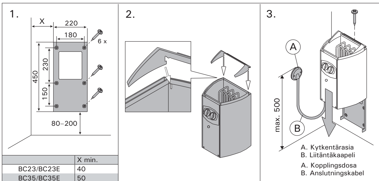
Kuva 7. Kiukaan kiinnittäminen seinään (mitat millimetreinä)
