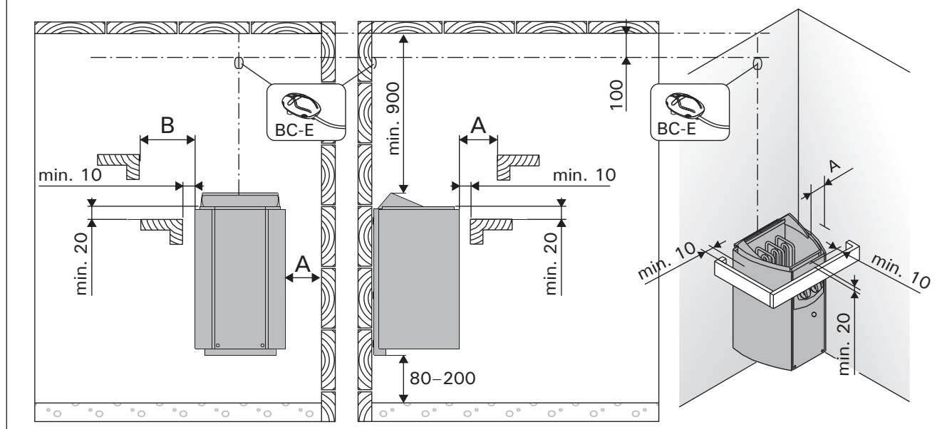
Рисунок 6. Расстояния безопасности (все размеры приведены в миллиметрах) Joonis 6. Kerise ohutuskaugused (kõik mõõtmised millimeetrites)
