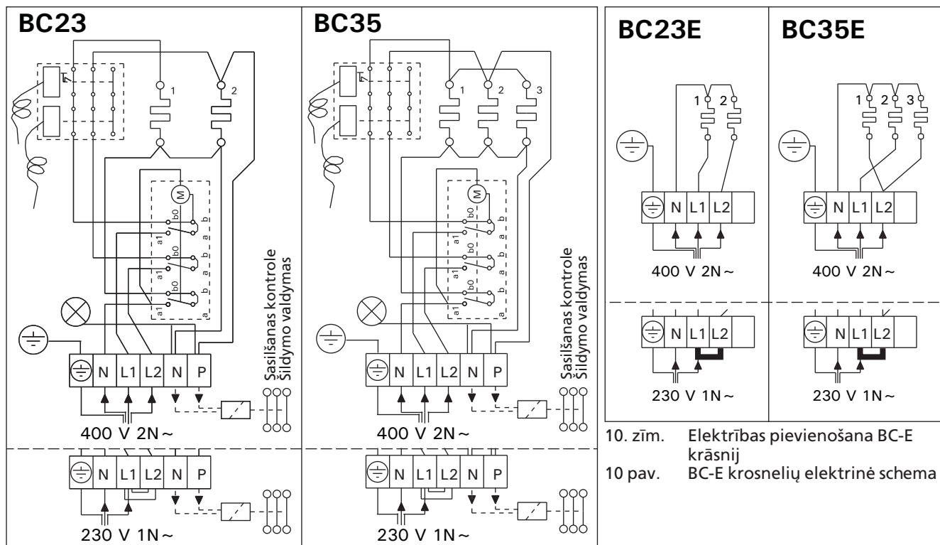
9. zīm. Elektrības pievienošana BC krāsnij 9 pav. BC krosnelių elektrinė schema
