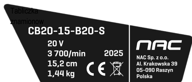
Tabliczka znamionowa
