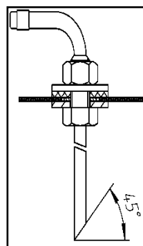
Rys. 19a – Instalacja wężyka ssącego paliwo
