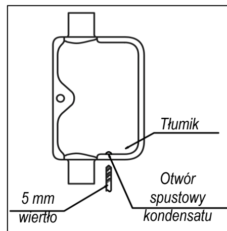
Rys. 14b. Otwór spustowy kondensatu przy montażu pionowym.
