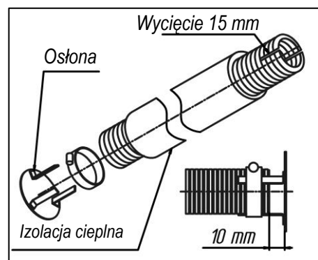
Rys. 13. Osłona rury wydechowej.
