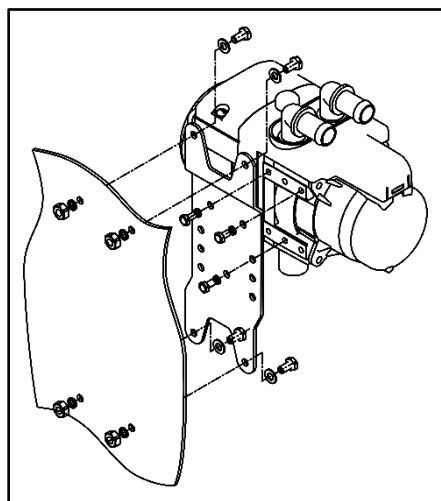
Rys. 2 - Montaż FLOW 5
