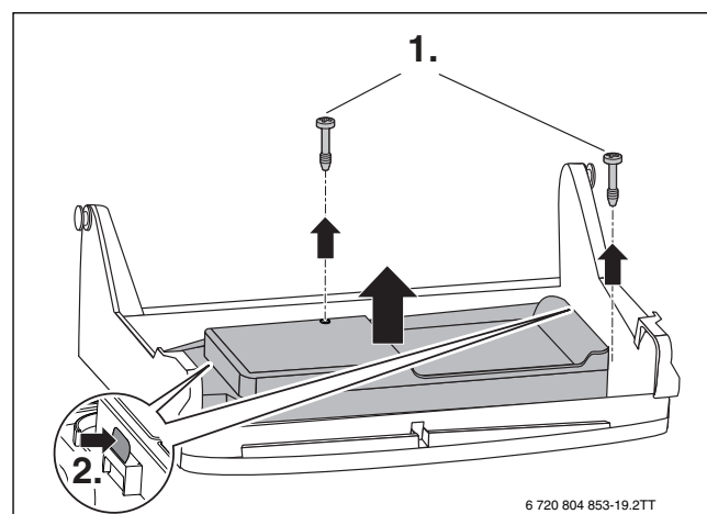
Rys. 71 Zdjęcie pokrywy
