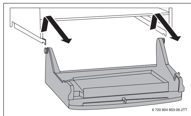
Rys. 72 Wyczepienie sterownika
