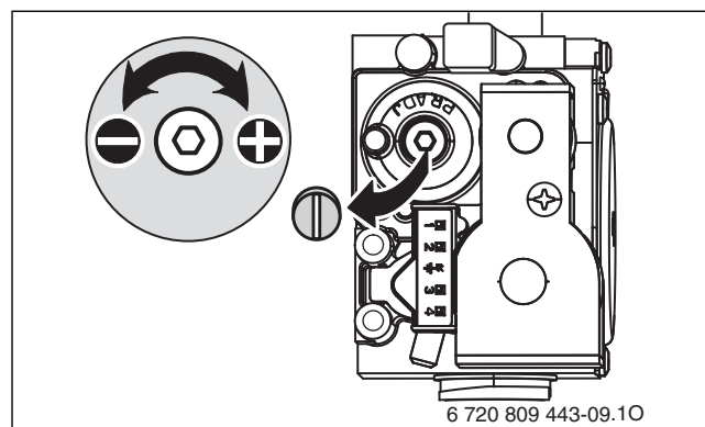
Rys. 43 Zdjąć plombę armatury gazowej
