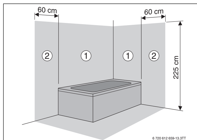
Rys. 27 Strefy ochronne
