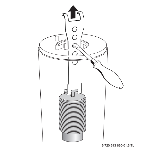
Rys. 53 Wyjmowanie dolnego elementu waporowego
