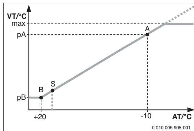
Rys. 79 Krzywa grzewcza
