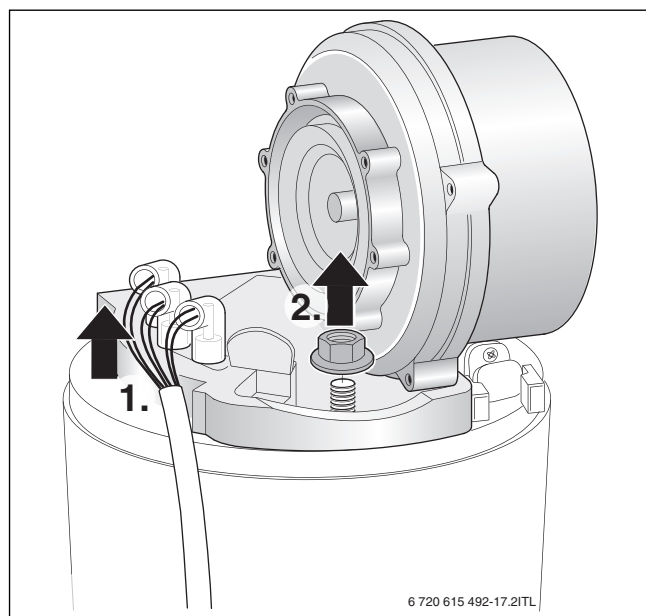
Rys. 50 Wyjmowanie wentylatora
