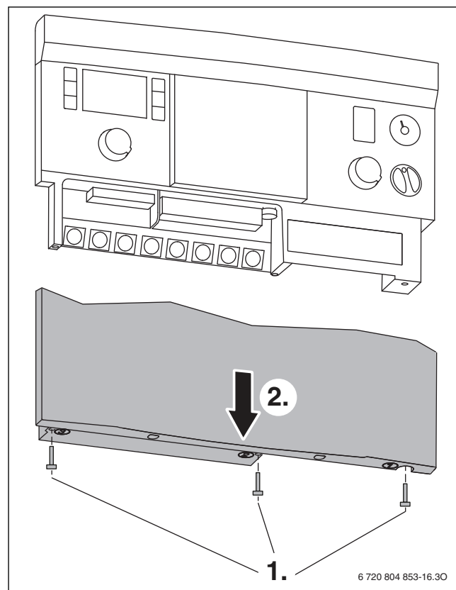
Rys. 30 Zdjęcie pokrywy
