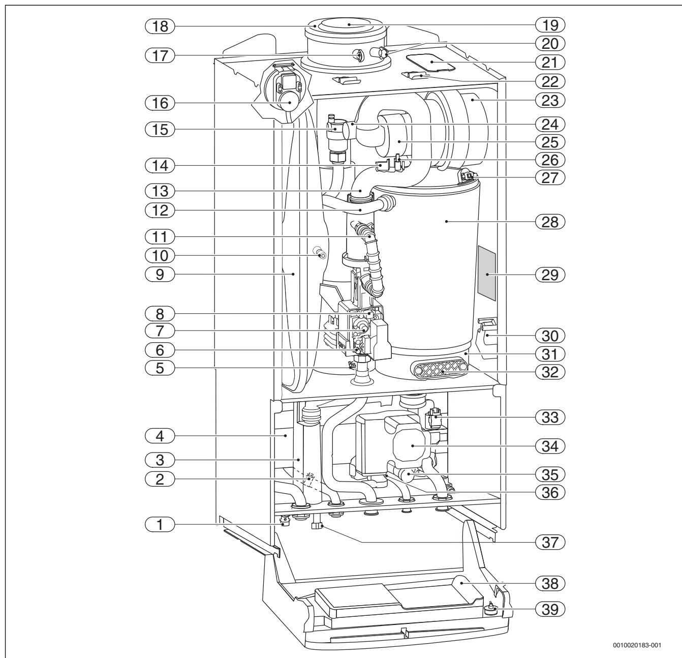
Rys. 3 Przegląd produktu
