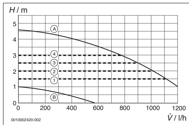
Rys. 80 Charakterystyki wykreślnie pompy i charakterystyki pompy
