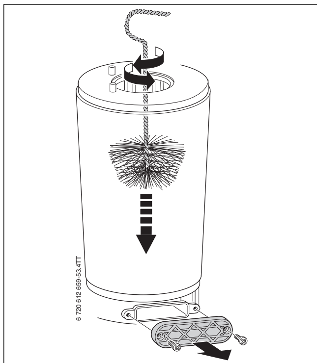
Rys. 54 Czyszczenie wymiennika ciepła
