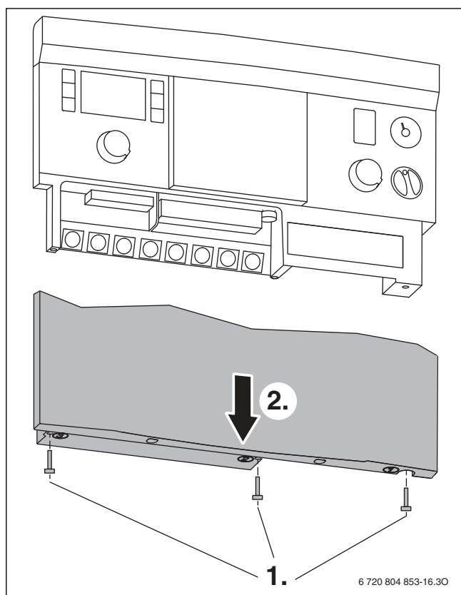
Rys. 69 Zdjęcie pokrywy
