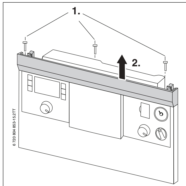
Rys. 28 Zdjęcie pokrywy
