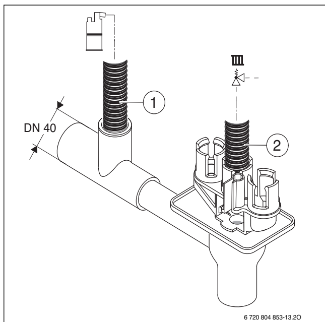
Rys. 25 Montaż węża kondensatu i węża zaworu bezpieczeństwa na syfonie
