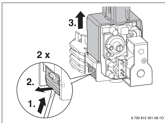
Rys. 67 Demontaż armatury gazowej
