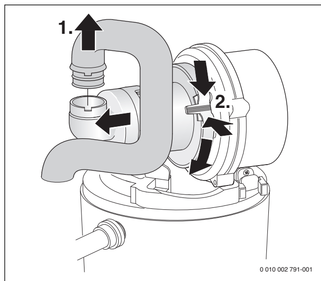
Rys. 49 Demontaż rury ssącej i urządzenia mieszającego
