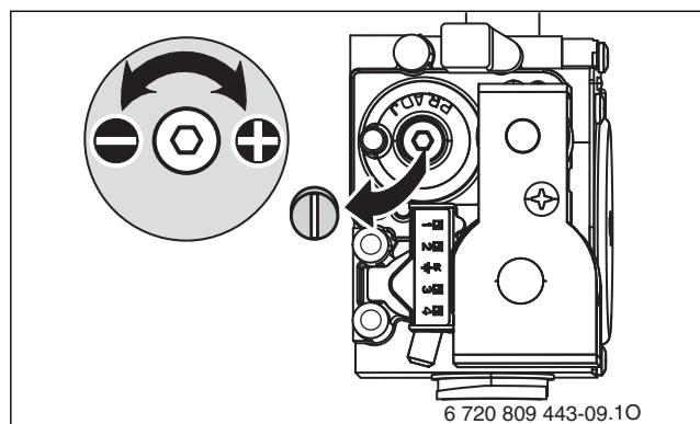
Rys. 38 Zdjęcie plomby armatury gazowej
