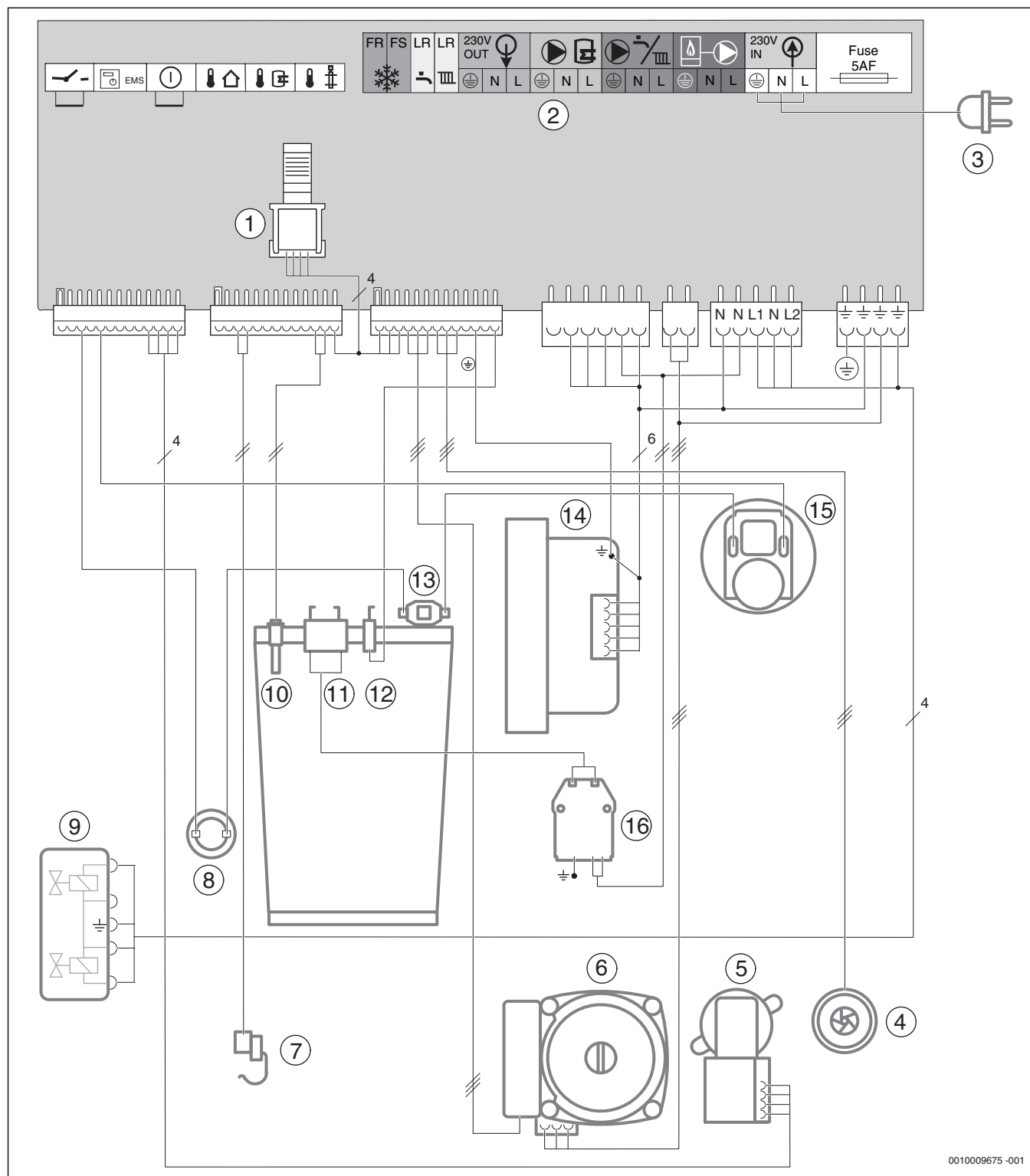
Rys. 78 Okablowanie elektryczne
