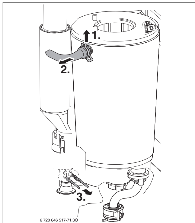
Rys. 73 Uwalnianie rury zasilającej i odłączanie kabla
