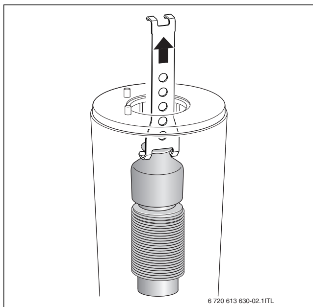
Rys. 52 Wyjmowanie górnego elementu waporowego
