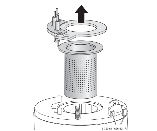
Rys. 51 Wyjmowanie palnika
