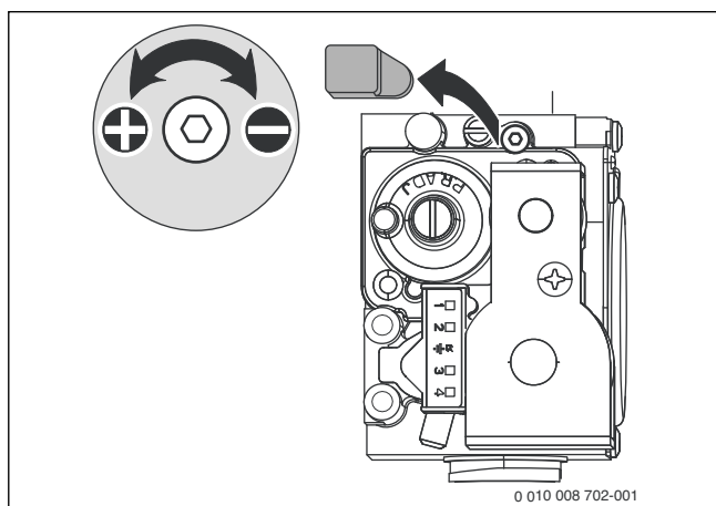
Rys. 41 Zdjąć plombę
