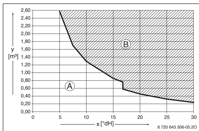
Rys. 20 Wymagania dotyczące wody do napełniania i uzupełniania w °dH do urządzeń o mocy < 50 kW
