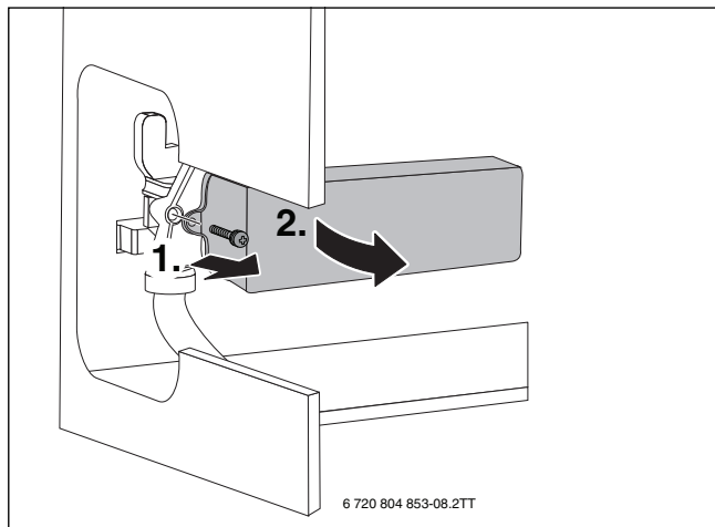
Rys. 61 Demontaż płytowego wymiennika ciepła
