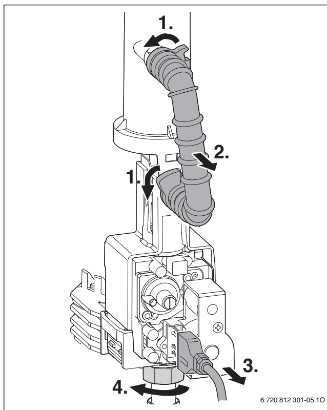
Rys. 66 Demontaż armatury gazowej
