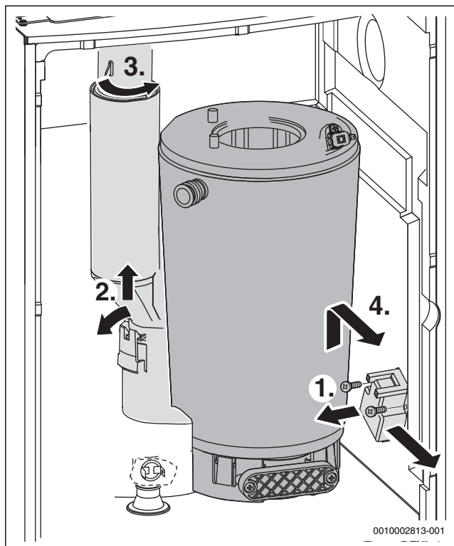
Rys. 75 Demontaż wymiennika ciepła
