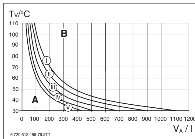
Rys. 22 Krzywe charakterystyczne wielkości naczynia wzbiorczego
