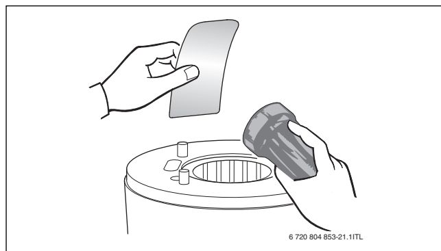
Rys. 55 Sprawdzenie wymiennika ciepła pod kątem pozostałości
