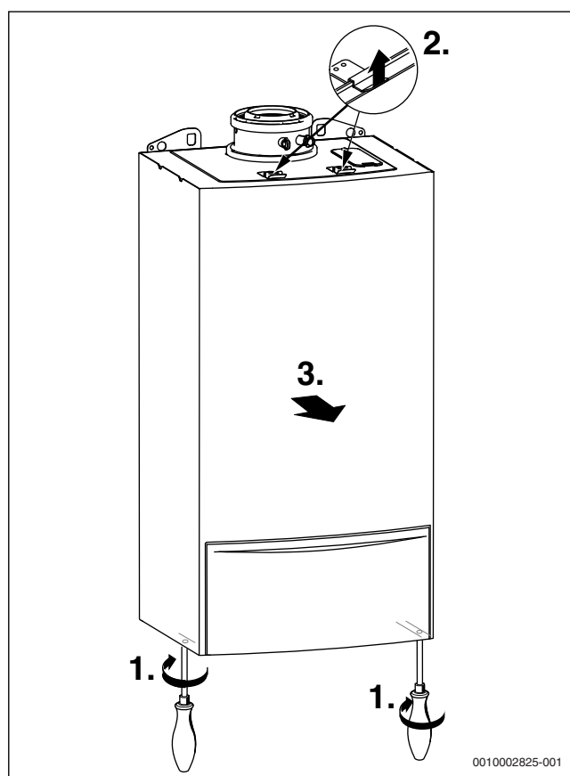
Rys. 23 Zdejmowanie obudowy
