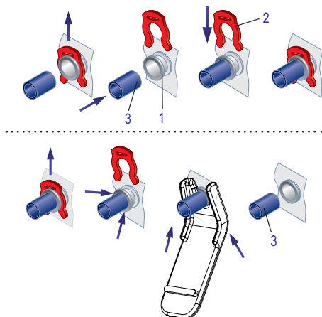
Rys. 7. Podłączenie wężyków
