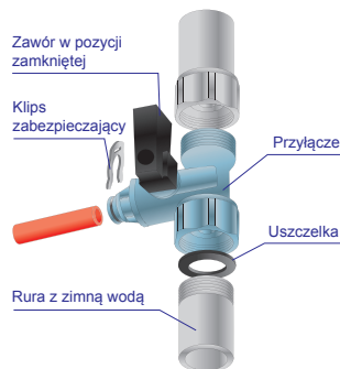
Rys.3. Przyłączy wody
