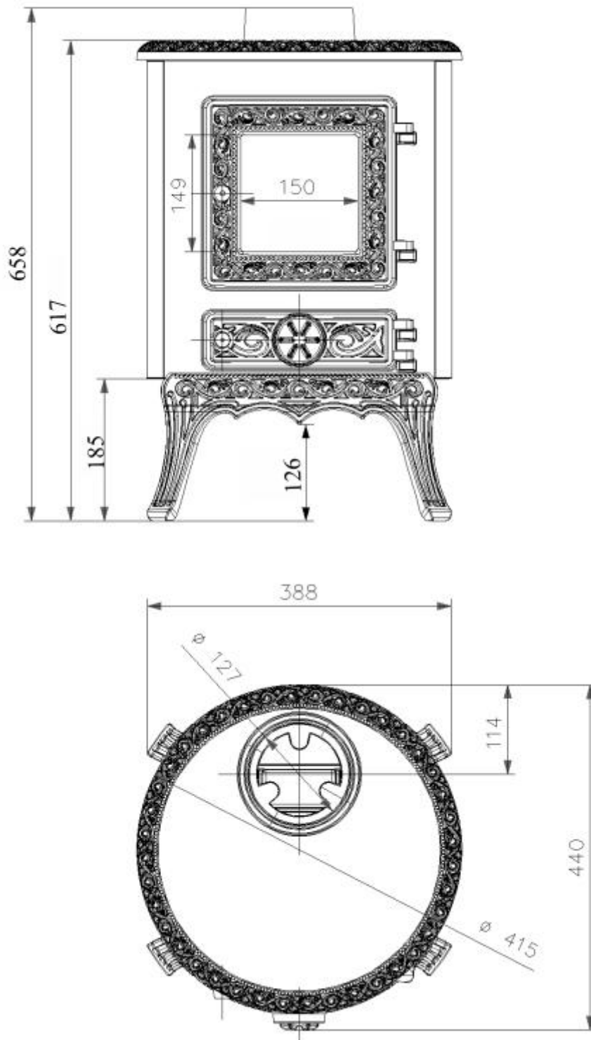
Rys. 1. [PL] Wymiary gabarytowe/ [CZ] Rozměry/ [HU] Befoglaló méreték/ [SK] Objemové rozmery/ [EN] Overall dimensions/ [LT] Gabaritiniai matmenys/ [LV] Vispārējie izmēri/ [RU] Габаритные размеры/ [EE] Üldmõõtmed/ [GR] Συνολικές διαστάσεις/ [RO] Dimensiuni gabarit/ [BG] Габаритни размери/ [UA] Габаритні розміри/ [NL] Productafmetingen/ [HR] Ukupne dimenzije/ [TR] Boyutlar/ [PT] Dimensões gerais/ [FR] Dimensions hors tout/ [ES] Dimensiones totales
