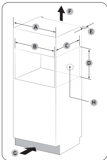
Dulap încadrat (mm)
