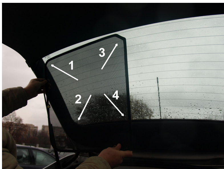
Rys.6 - Montaż zasłonek klapy bagażnika
