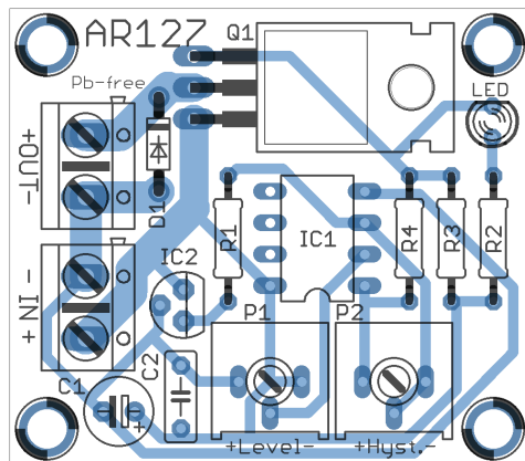
Rys. 2 Schemat montażowy
