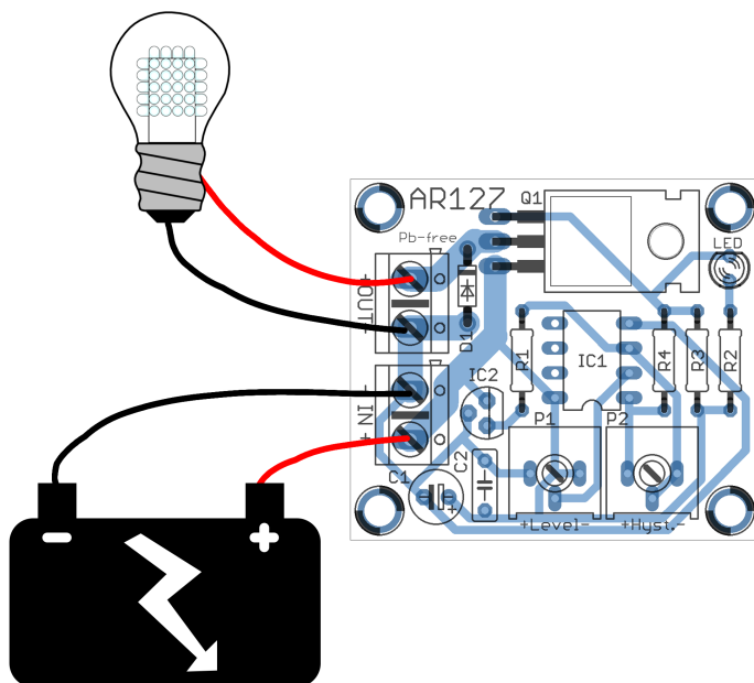
Rys. 3 Przykład podłączenia
