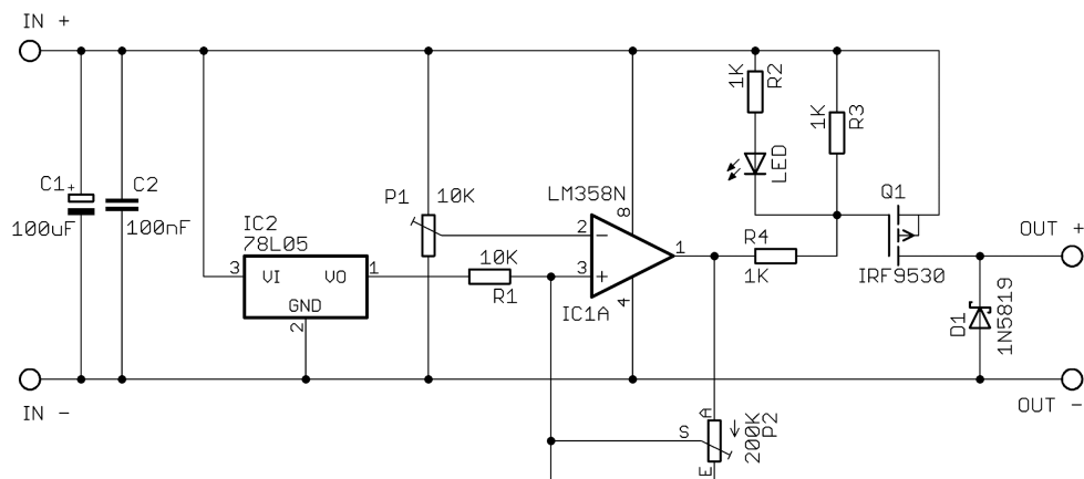
Rys. 1 Schemat ideowy
