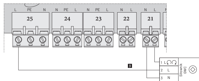
Rys. Schemat podłączenia przepustnicy iZZi GWC
