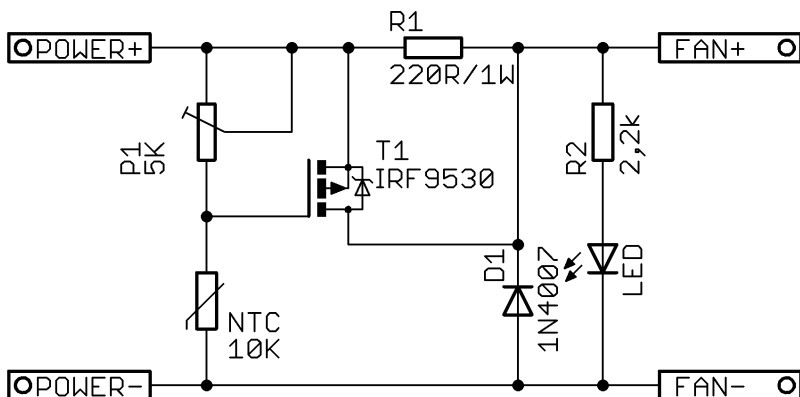
Rys. 2 Schemat ideowy
