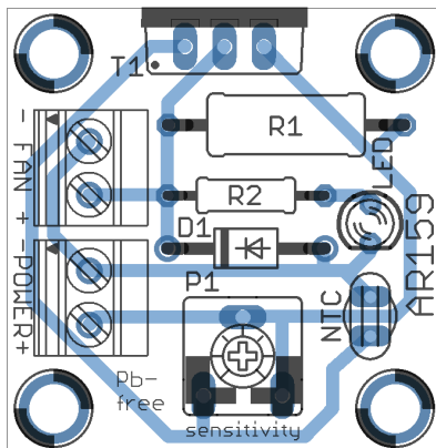
Rys. 1 Schemat montażowy
