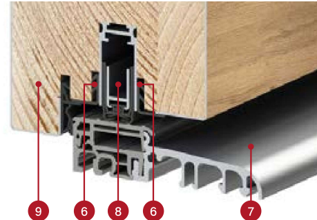
przekrój skrzydła THERMO 78 z uszczelką i bez uszczelki opadającej, próg aluminiowy
