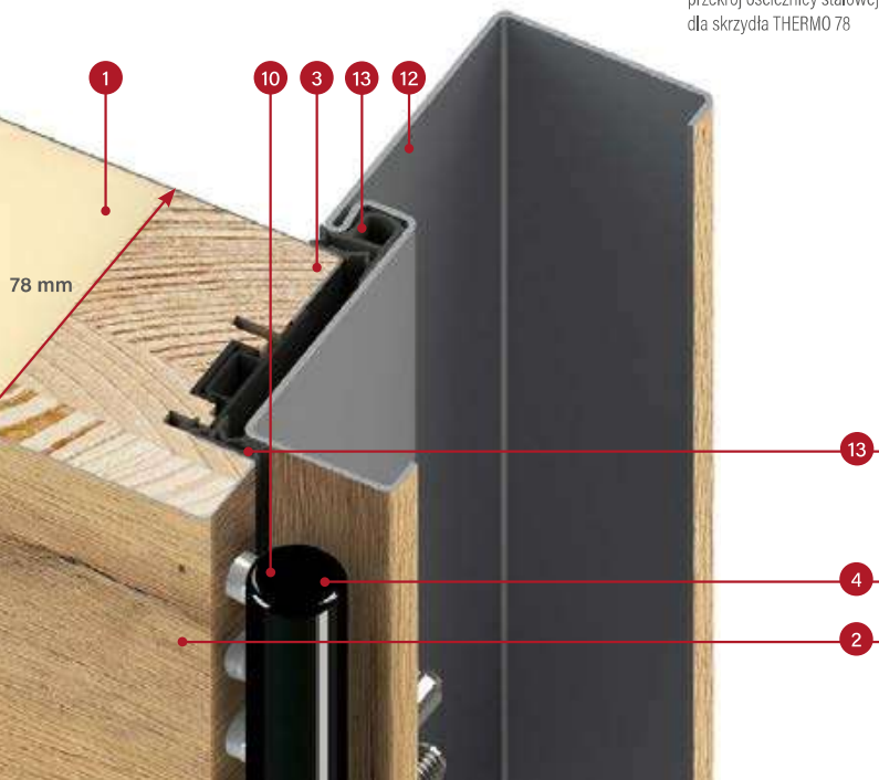
przekrój ościeznicy stalowej dla skrzydła THERMO 78
