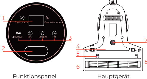
Funktionspanel
