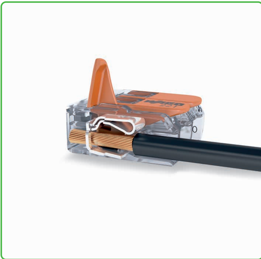
Oprzewodowanie puszki instalacyjnej przy użyciu przewodów linkowych
