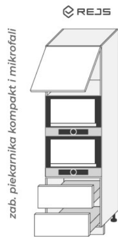
D14 RU 2R KOMPAKT (600/2070/565)
