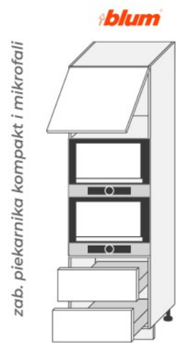
D14 RU 2M KOMPAKT ● (600/2070/565)
