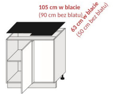
D13U 90 L/P (900/820/500)
