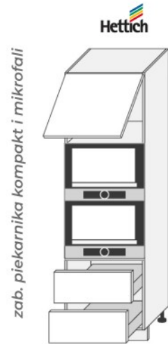
D14 RU 2A KOMPAKT (600/2070/565)
