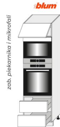
D14 RU 2M 60 284 ● (600/2070/565)
