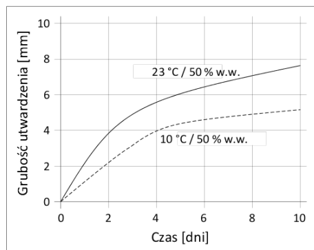
Wykres 1: Szybkość utwardzania Sikaflex®-521 UV
