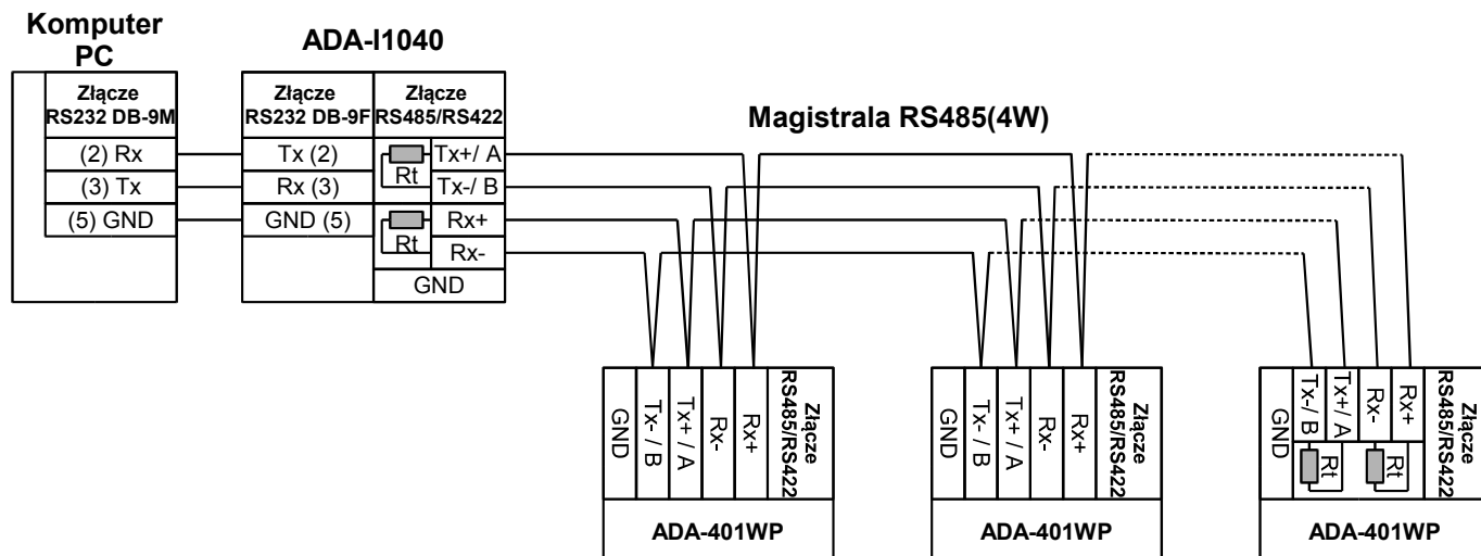
Rys 3. Przykładowe podłączenie modułów ADA-401WP do 4-przewodowej magistrali RS485
