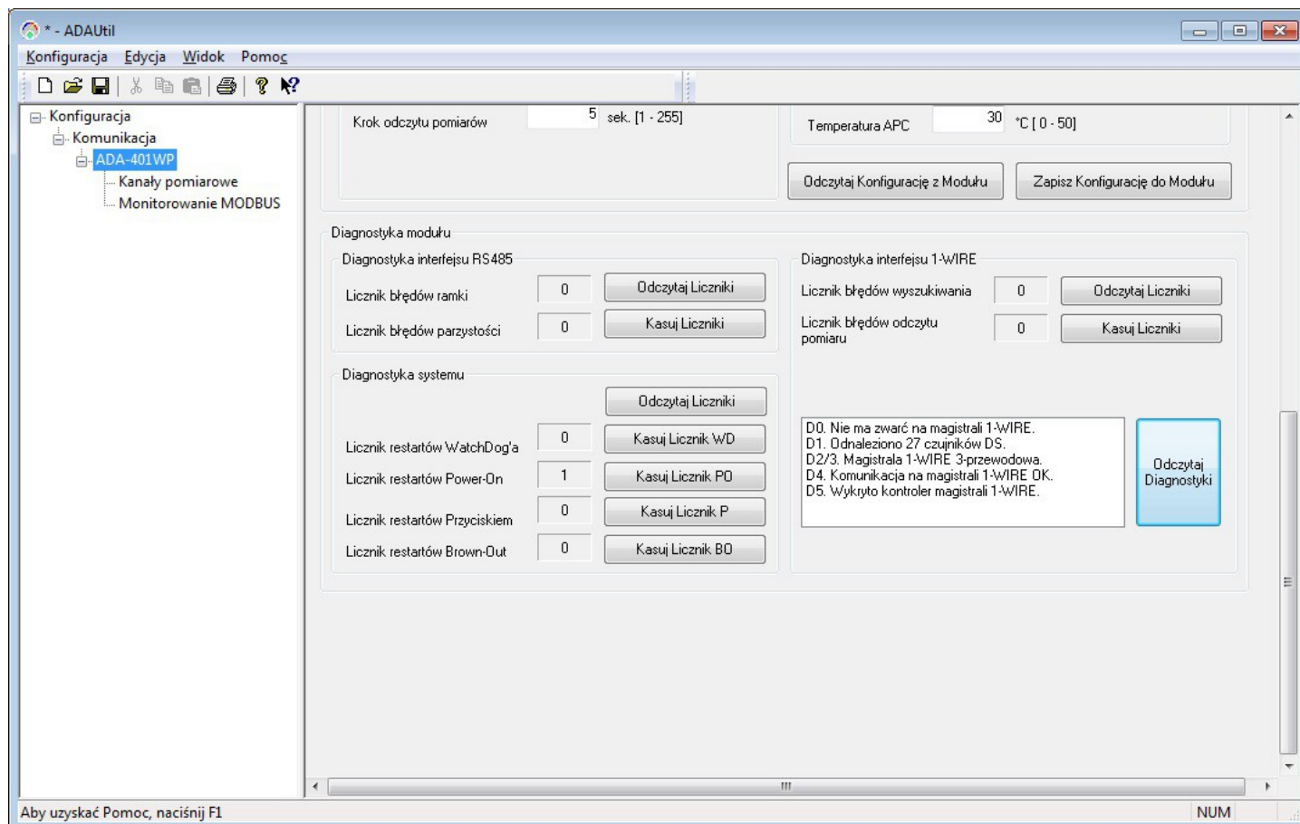
Rys 11. Widok diagnostyki głównej modułu w programie ADAUtil
