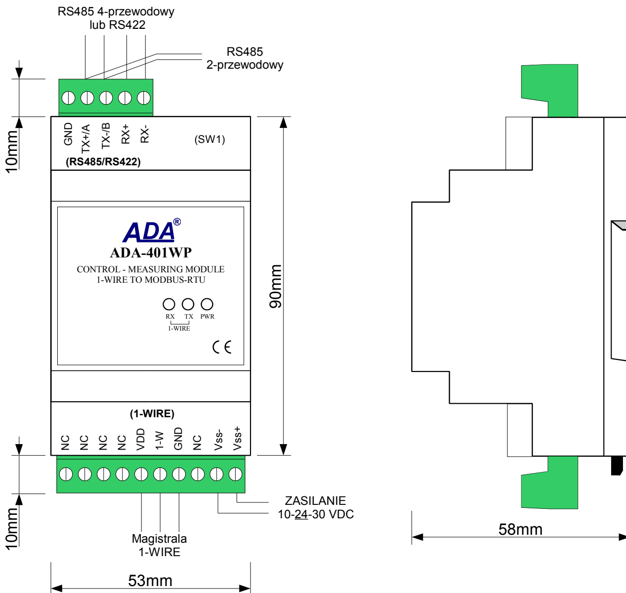
Rys. 1. Widok ADA-401WP
