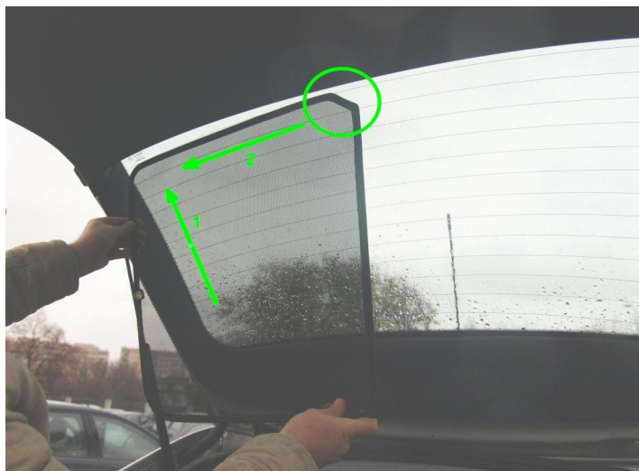
Zdjęcie nr 6 - Montaż zasłonek klapy bagażnika
