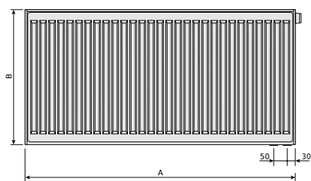
Ventil Compact, prawy, widok z przodu
