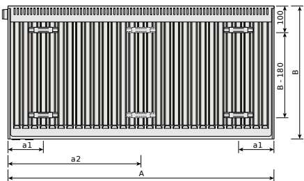
Ventil Compact, typ 11, widok z tyłu
