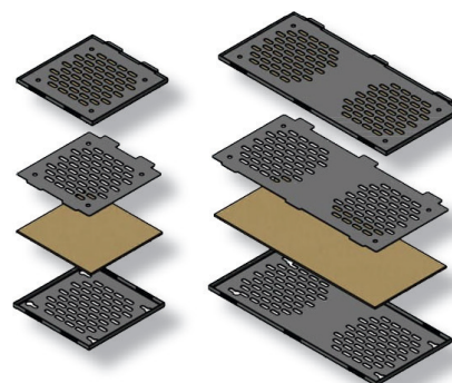
Kaseta filtracyjna (nr kat. KF-1-S lub KF-2-S)
