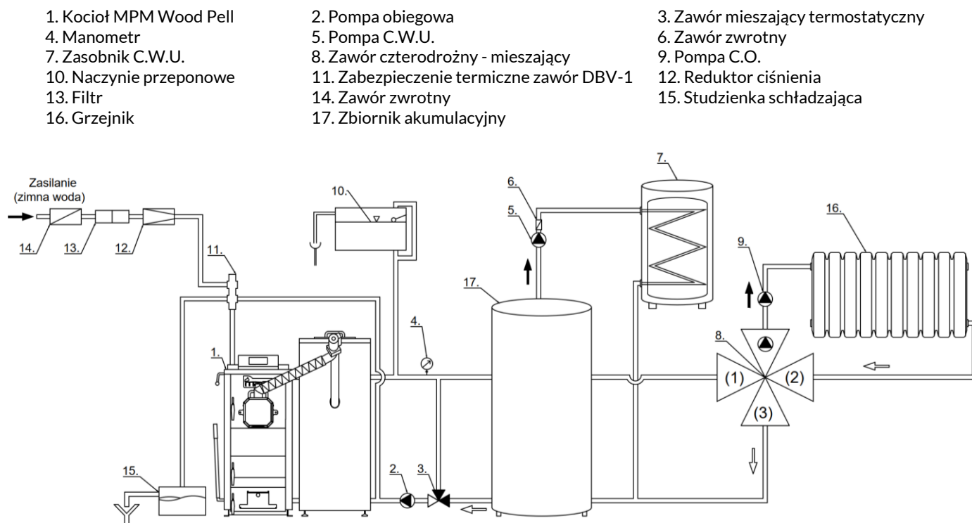
Rysunek 3. Przykładowy schemat podłączenia kotła MPM Wood Pell w układzie otwartym.
