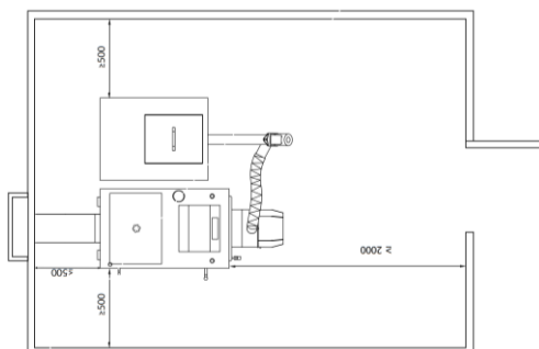
Rysunek 5. Ustawienie kotła w pomieszczeniu kotłowni.
