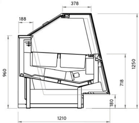
Sezione Section H 1250
