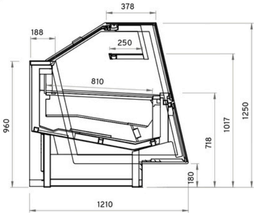
Sezione Section H 1250
