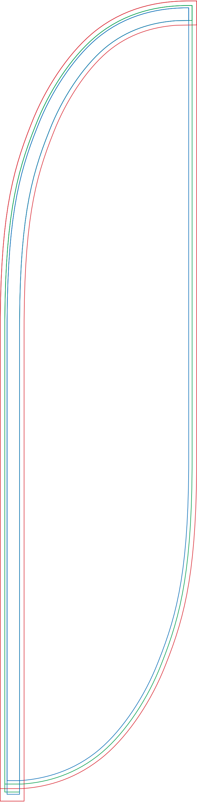
Bowflag®100 L ( wypukły ) 80 x 340 cm wymiar z naddatkami: 86,5 x 352 cm
