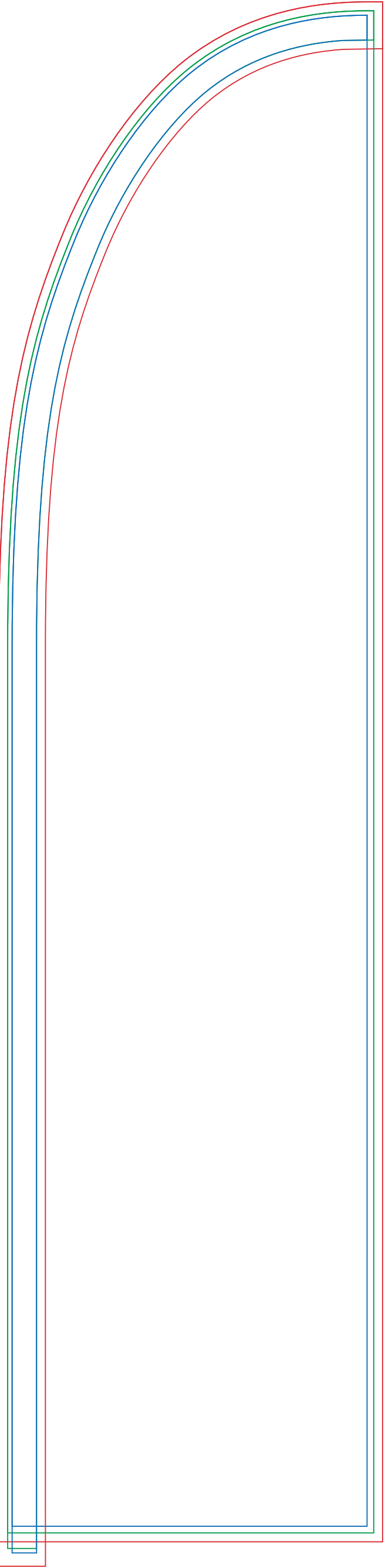
Bowflag®100 L ( prosty ) 80 x 340 cm wymiar z naddatkami: 86,5 x 352 cm
