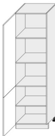
D14 DP 60 (600/2070/565)
