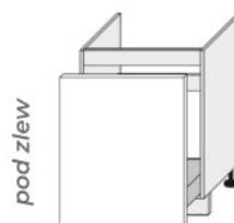
D1ZA 60 (600/820/500)
