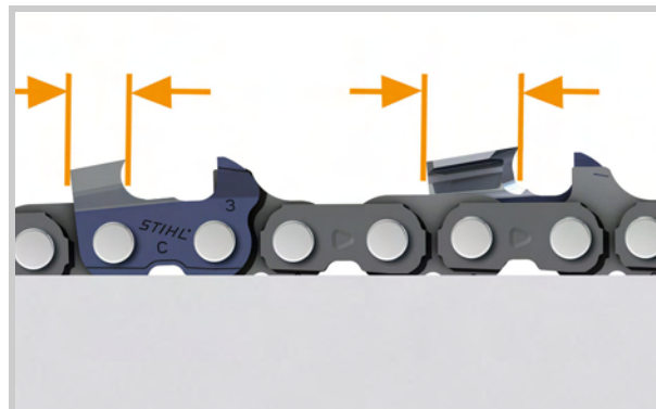
Różne długości zębów
