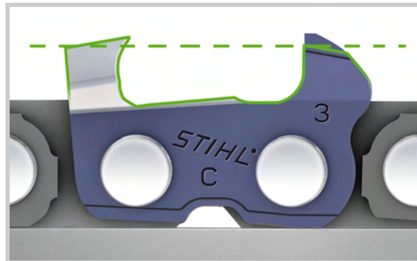
Za mały odstęp ogranicznika zagłębienia
