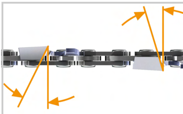
Różne kąty ostrzenia
