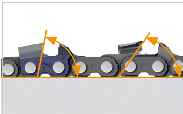
Różne kąty natarcia
