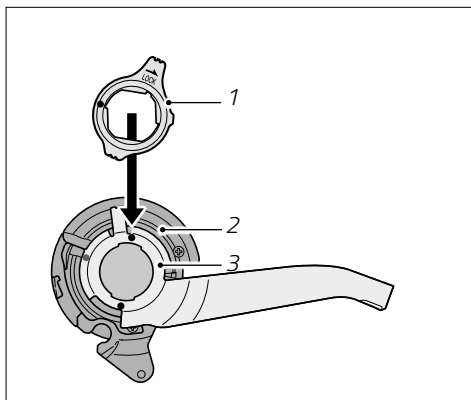
Rys.: Komponenty przerzutki wewnętrznej (przekład)
