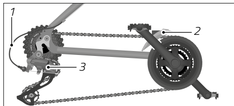
Rys.: Komponenty przerzutki zewnętrznej (przykład)
