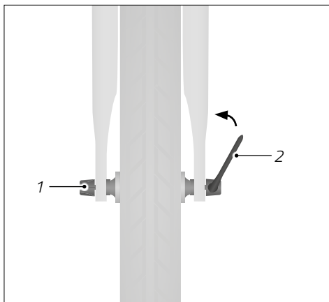
Rys.: Koło z osią szybkomocującą (przykład)
