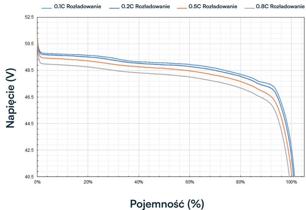
Krzywa stopnia rozładowania pod różnym napięciem poniżej 25°C
