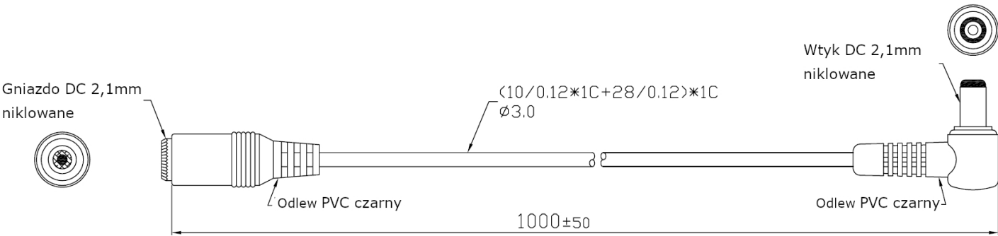
Schemat połączeniowy
