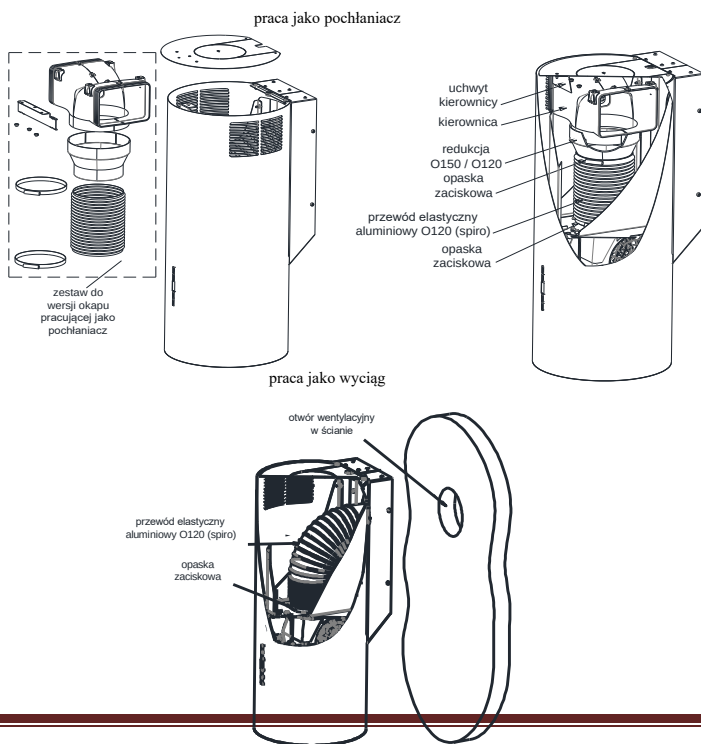
Rys. 3 Opcje montażu: pochłaniacz lub wyciąg
