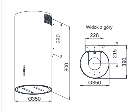
Rys. 2 Rysunek gabarytowy.
