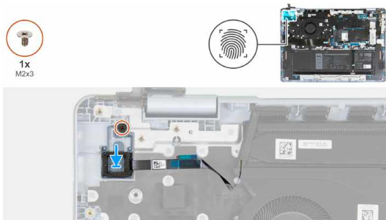
Rysunek 39. Instalowanie przycisku zasilania z opcjonalnym czytnikiem linii papilarnych
