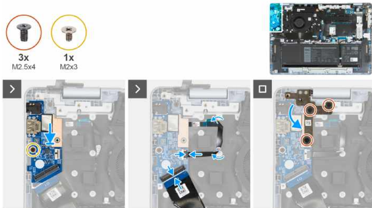
Rysunek 35. Instalowanie płyty we/wy
