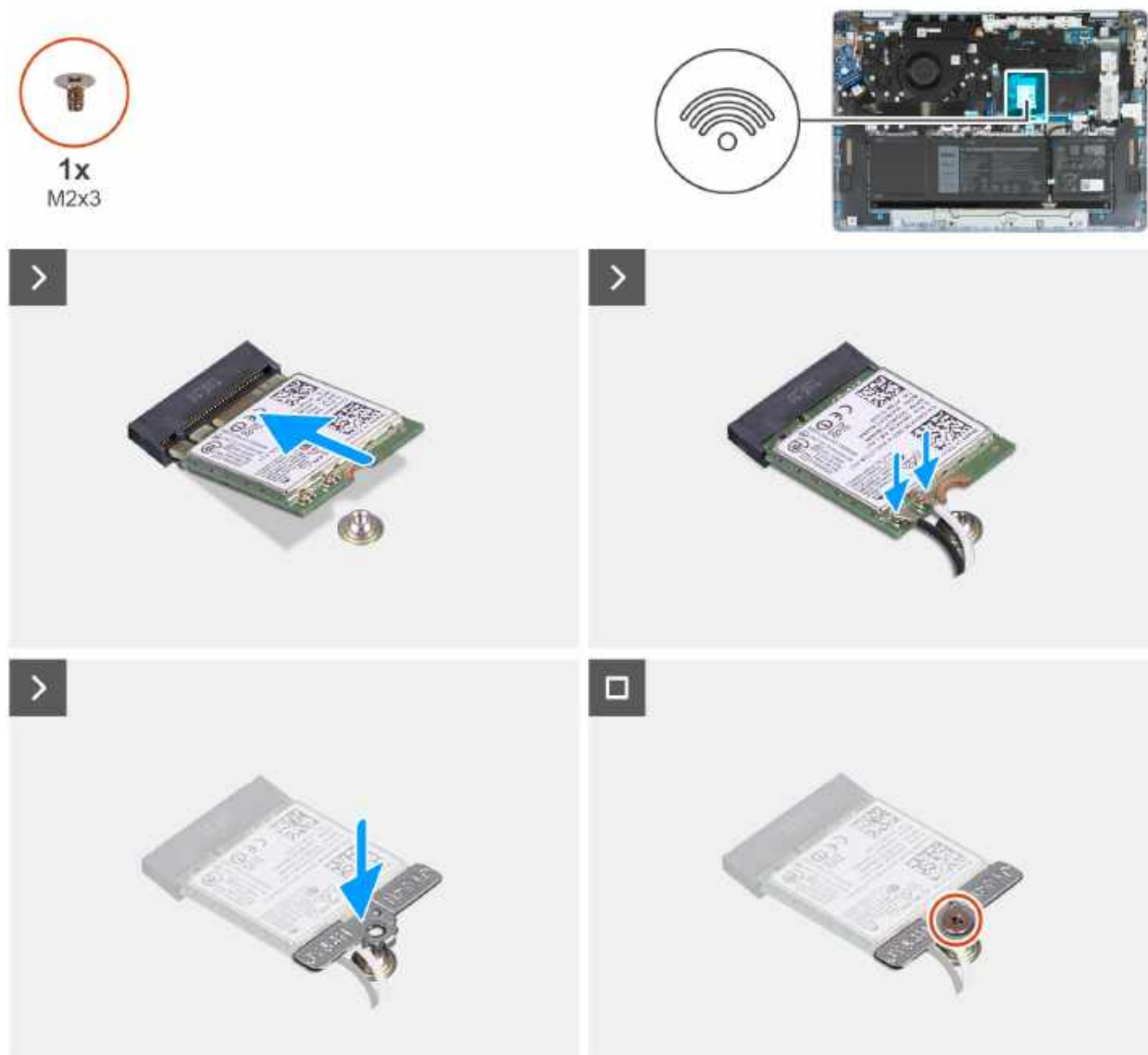
Rysunek 24. Instalowanie karty sieci bezprzewodowej
