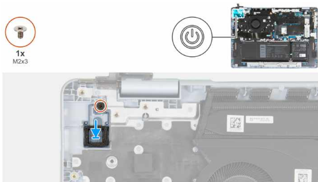
Rysunek 37. Instalowanie przycisku zasilania
