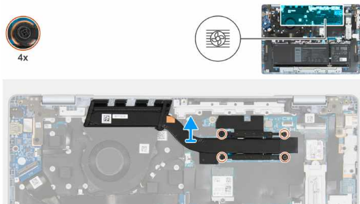
Rysunek 50. Wymontowywanie radiatora
