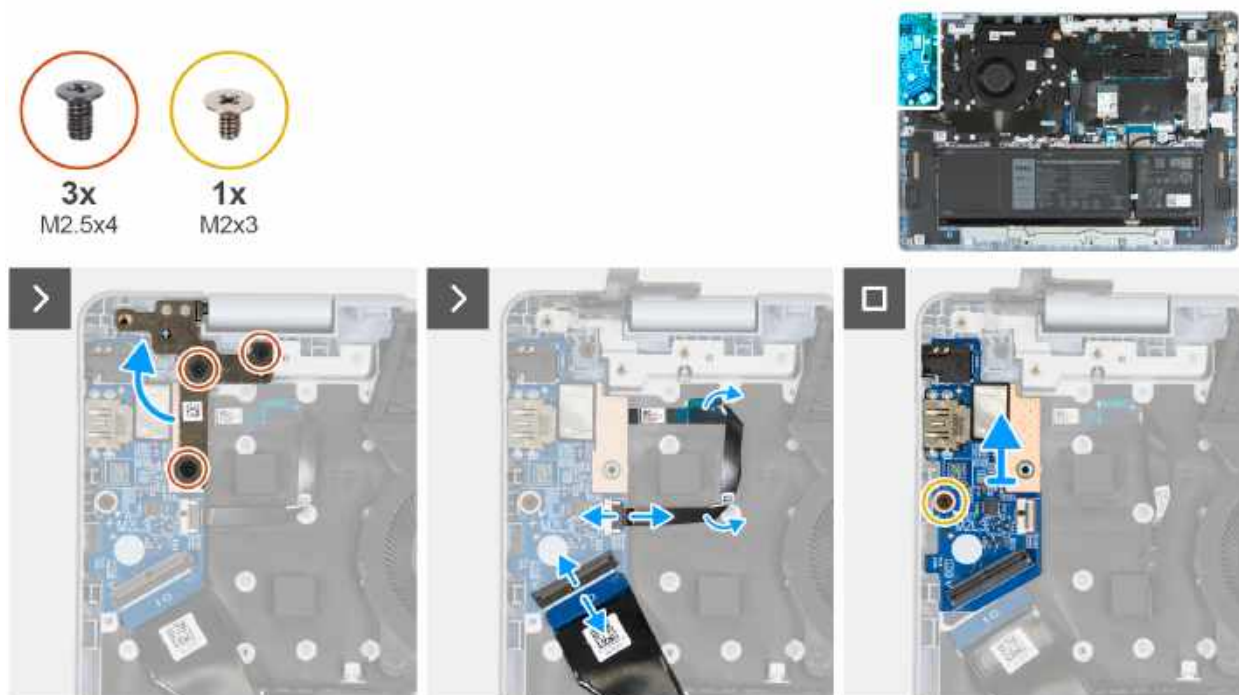
Rysunek 34. Wymontowywanie płyty we/wy
