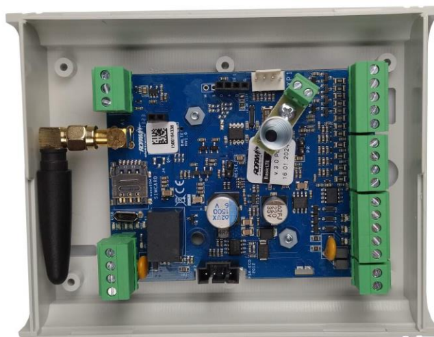
1 BasicLTE-BOX moduł w obudowie natynkowej z tamperem.
