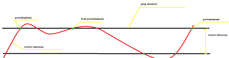
26 Graficzne przedstawienie histerezy.
