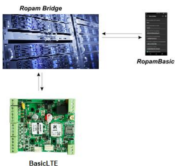
20 Schemat łączności pomiędzy modulem BasicLTE a aplikacją RopamBasic.
